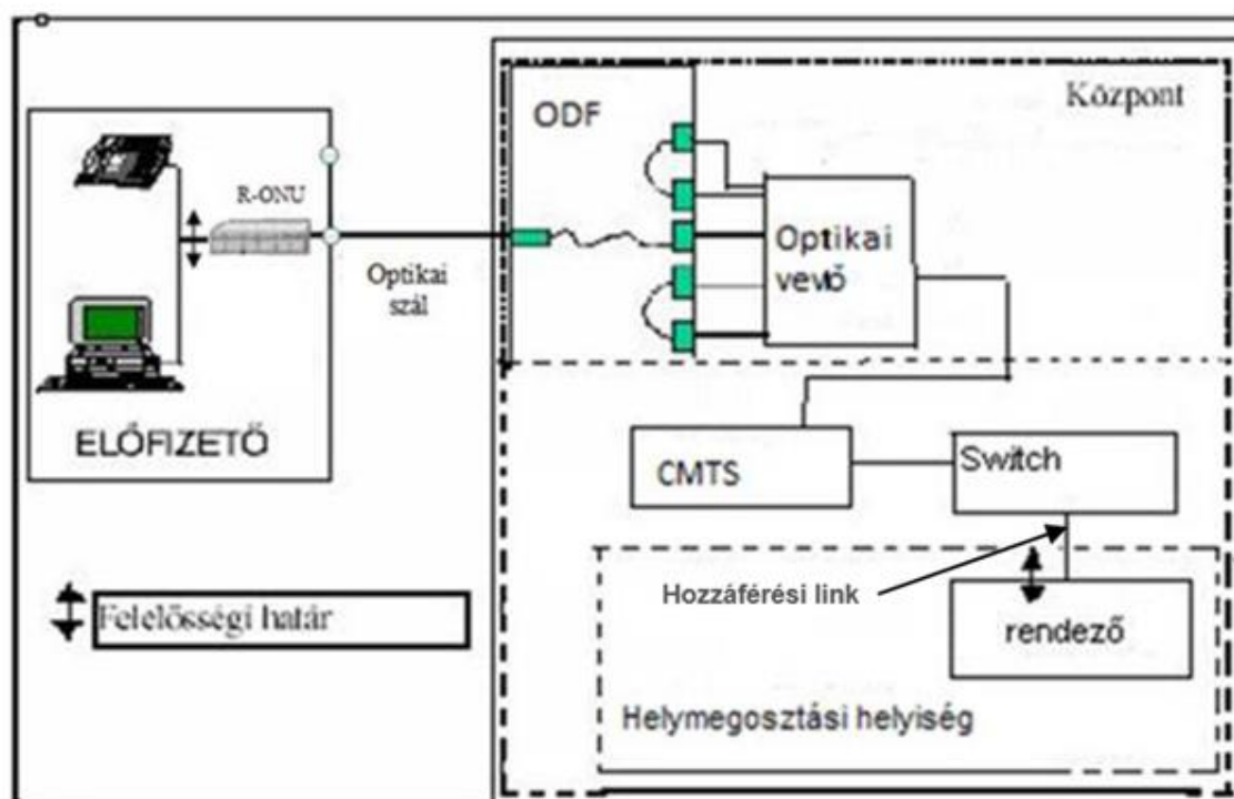
Közelitávközi Hozzáférés FTTH-RFoG Hozzáférési Hálózaton ábrája
